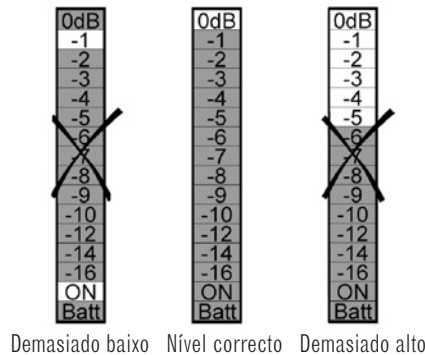
Figura 5. Ajustar os níveis do subwoofer para conseguir um pico de 0 dB
